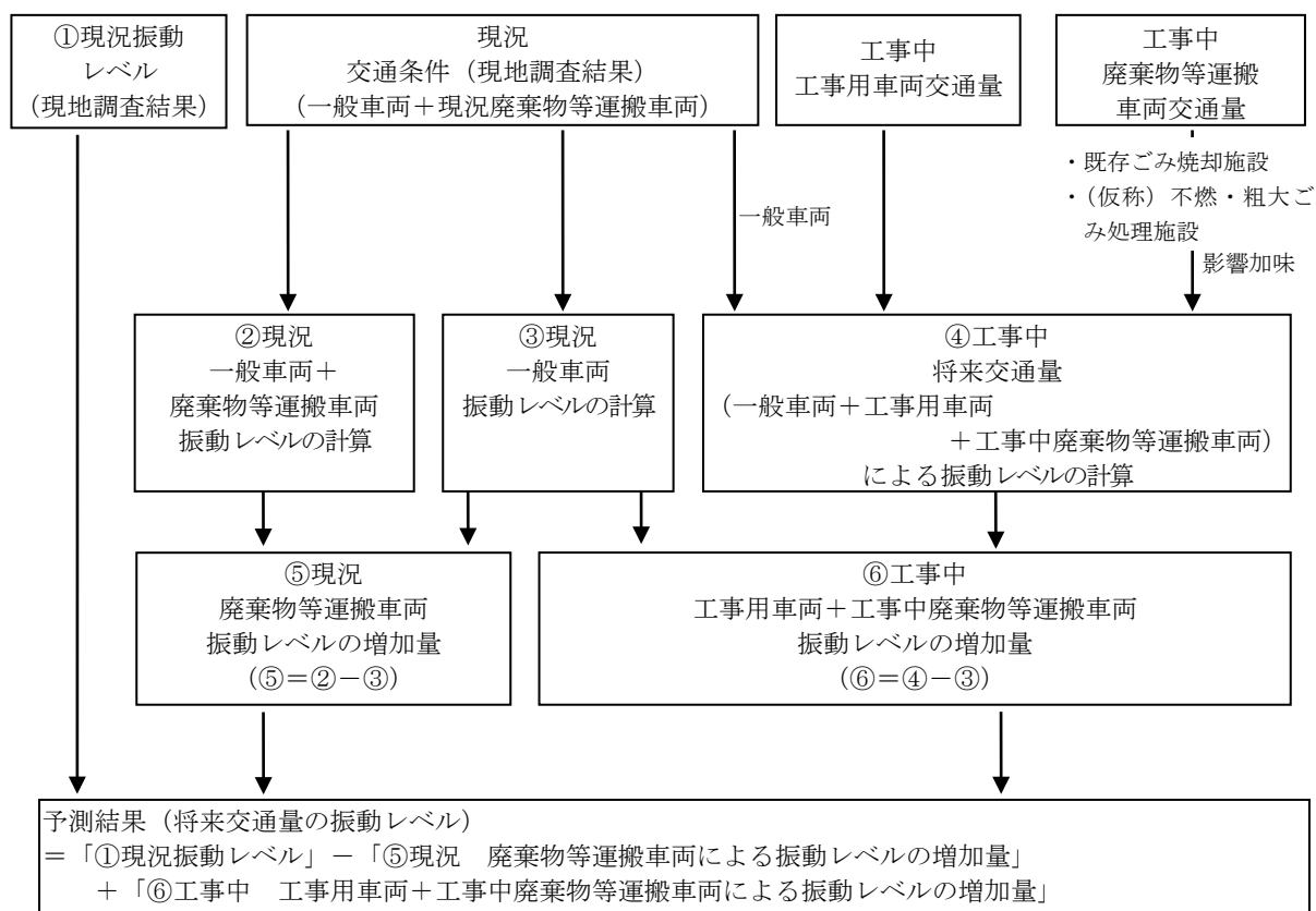
図 8.3-10 工事用車両の走行に伴う振動予測フロー
