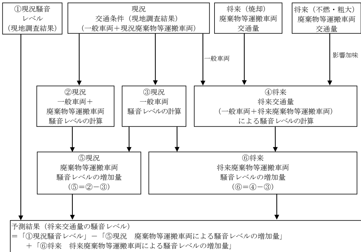
図 8.3-14 廃棄物等運搬車両の走行に伴う騒音予測フロー
