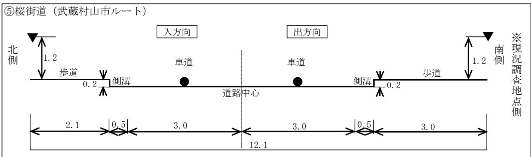
図 8.3-9 道路条件、音源位置図
