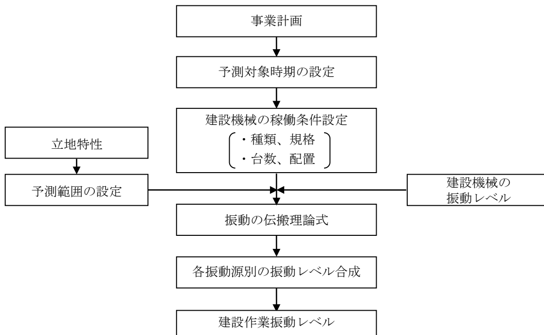
図8.3-7 建設機械の稼働に伴う振動予測フロー
