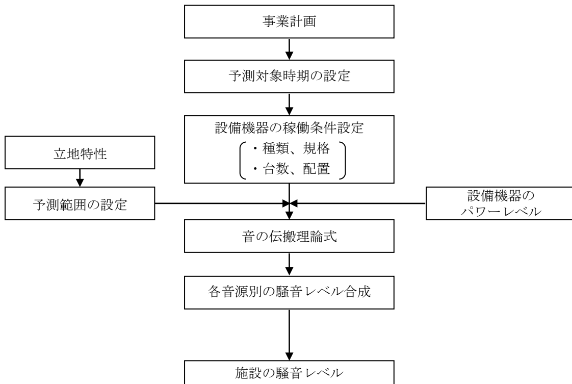
図8.3-12 施設の稼働に伴う騒音予測フロー
