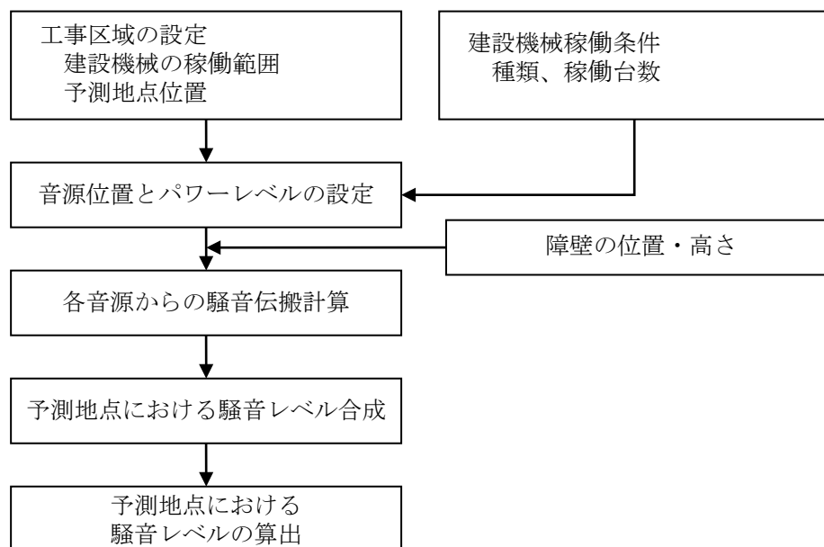
図 8.3-4 建設機械の稼働に伴う騒音予測フロー
