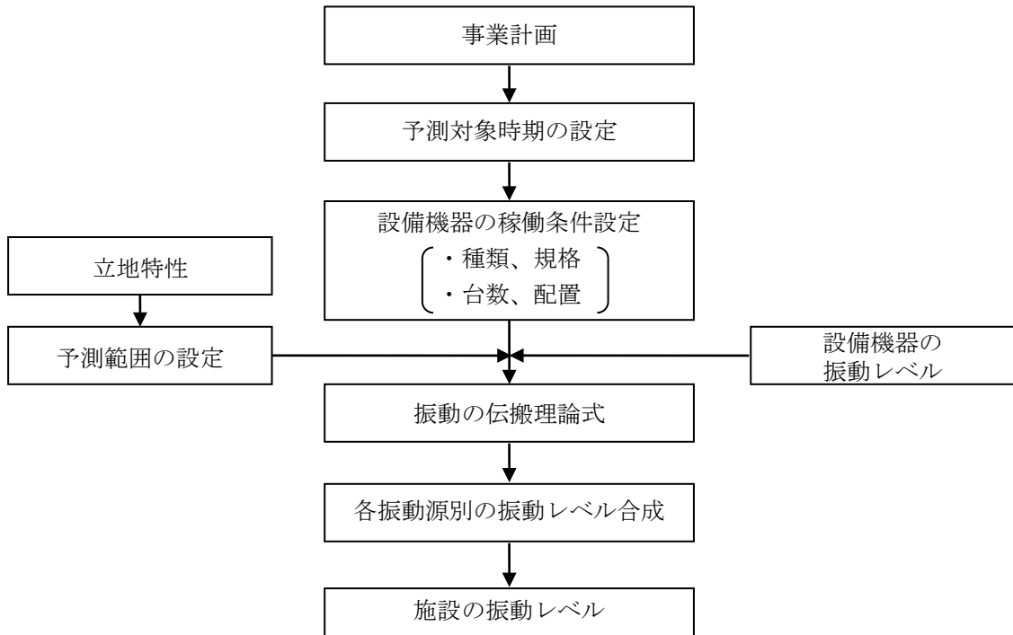
図8.3-13 施設の稼働に伴う振動予測フロー
