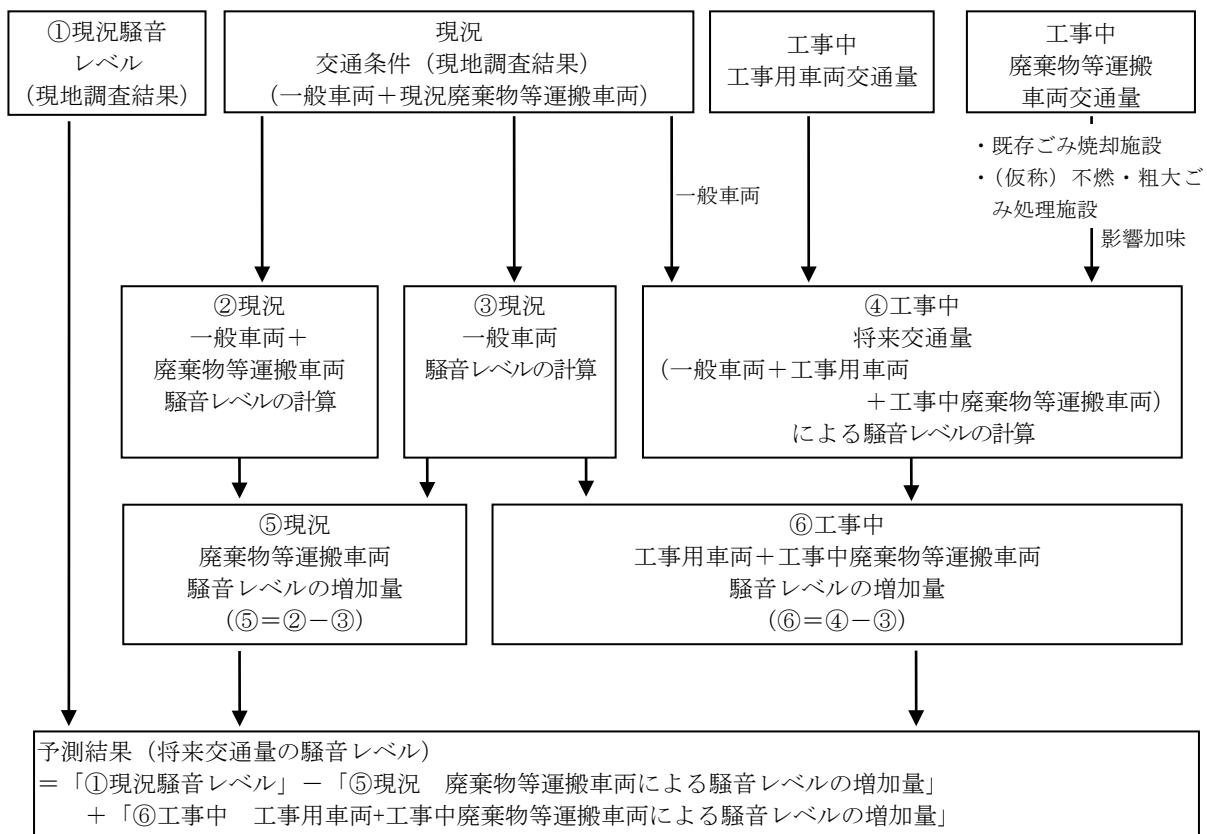
図 8.3-8 工所用車両の走行に伴う騒音予測フロー
